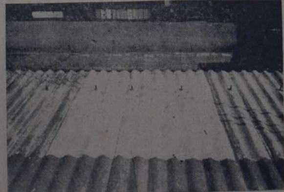
LA PRESENTE FOTOGRAFIA MUESTRA UNA CHAPA DE ZINC EX. puesta a los rigores del sol y la lluvia durante algún tiempo. La parte derecha ha sido pintada con albayalde puro y ya aparece completamente descolorida y protegida. La parte izquierda ha sido recubierta con pintura a base de plomo y se ve perfectamente la mancha oscura y venenosa.
